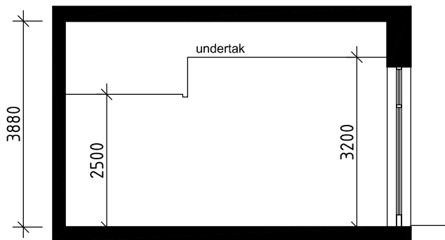
SEKTION A-A
