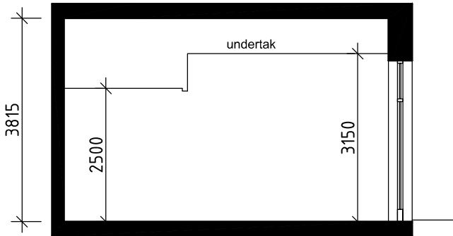
SEKTION A-A
