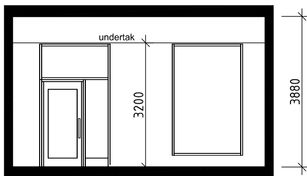
SEKTION B-B
