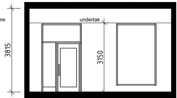
SEKTION B-B
