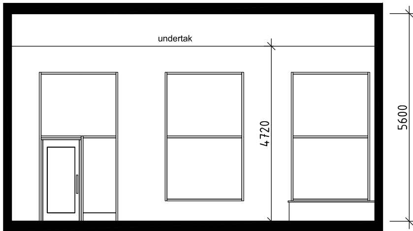
SEKTION A-A
