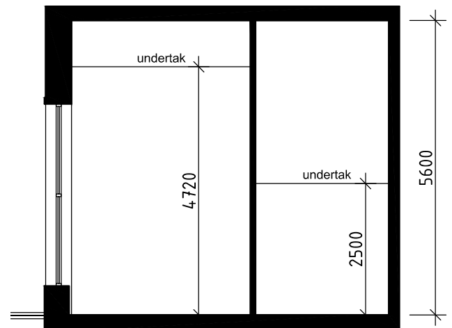
SEKTION B-B
