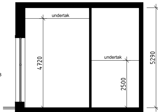
SEKTION B-B
