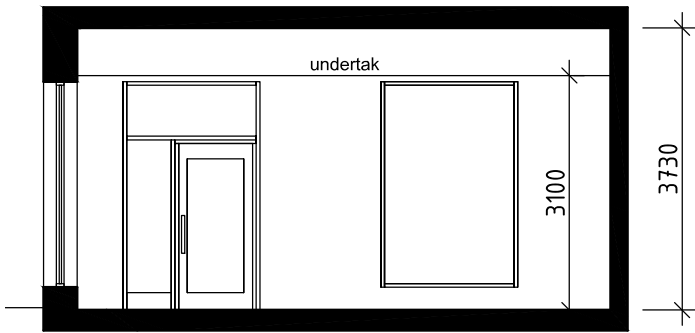
SEKTION A-A
