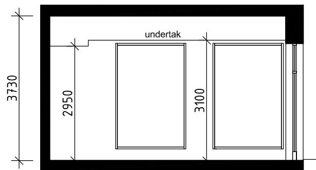
SEKTION C-C
